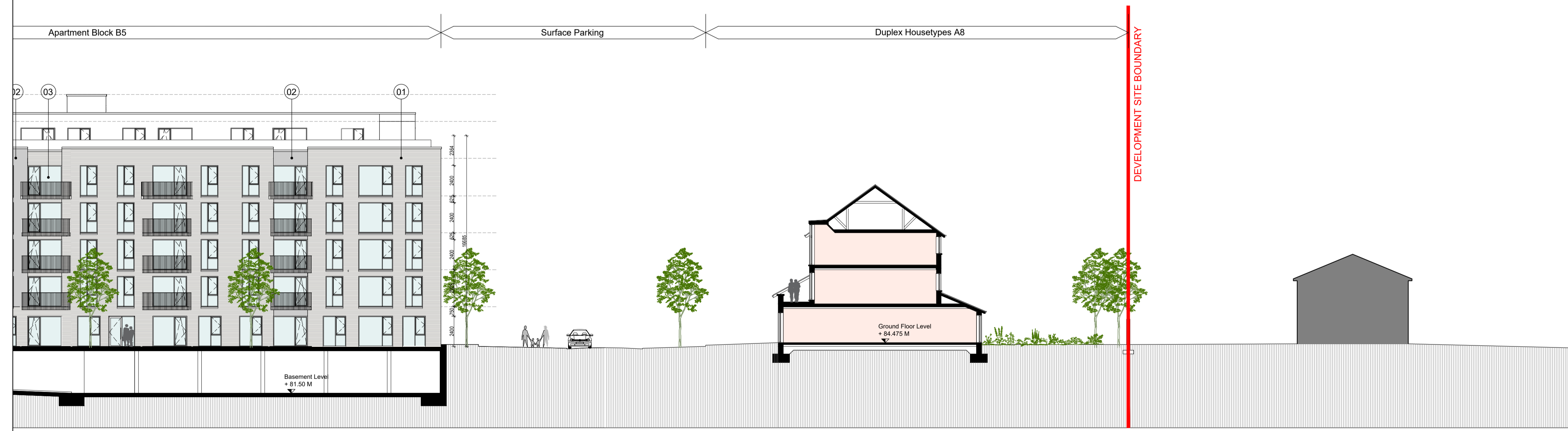
SITE SECTION C-C 1:200
